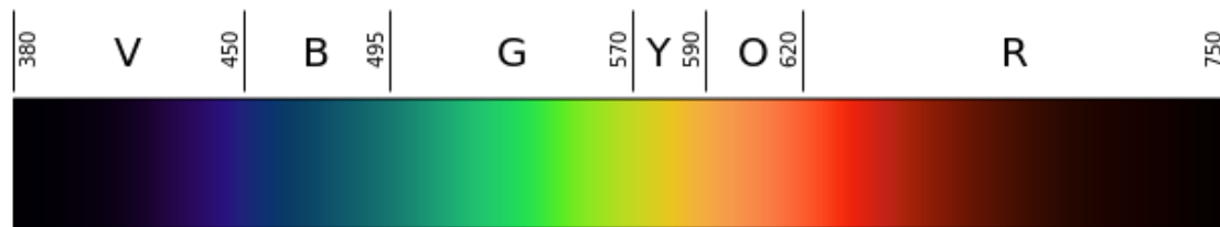
הספקטרום האלקטרומגנטי של התחום הנראה (380-750 nm).
