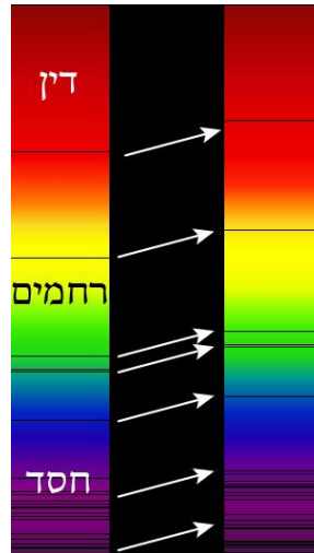
אור חוזר – הסטה לאדום
