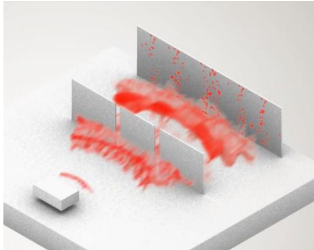
יורים גל של אור וכשהגל מגיע למסך אז הוא הופך להיות נקודה (חלקיק)
